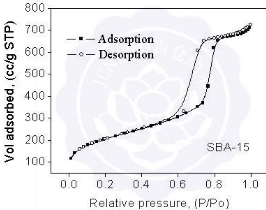
图 1-2 SBA-15 的氮气吸附等温线图[23]。
