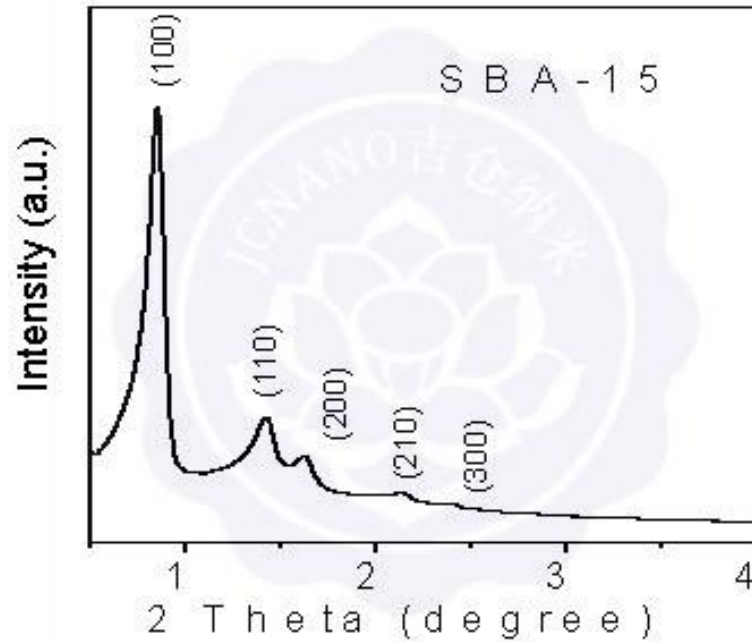
图 1-1 SBA-15 的小角 X 射线衍射图 (XRD) [23]。
